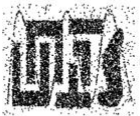
8000 points
